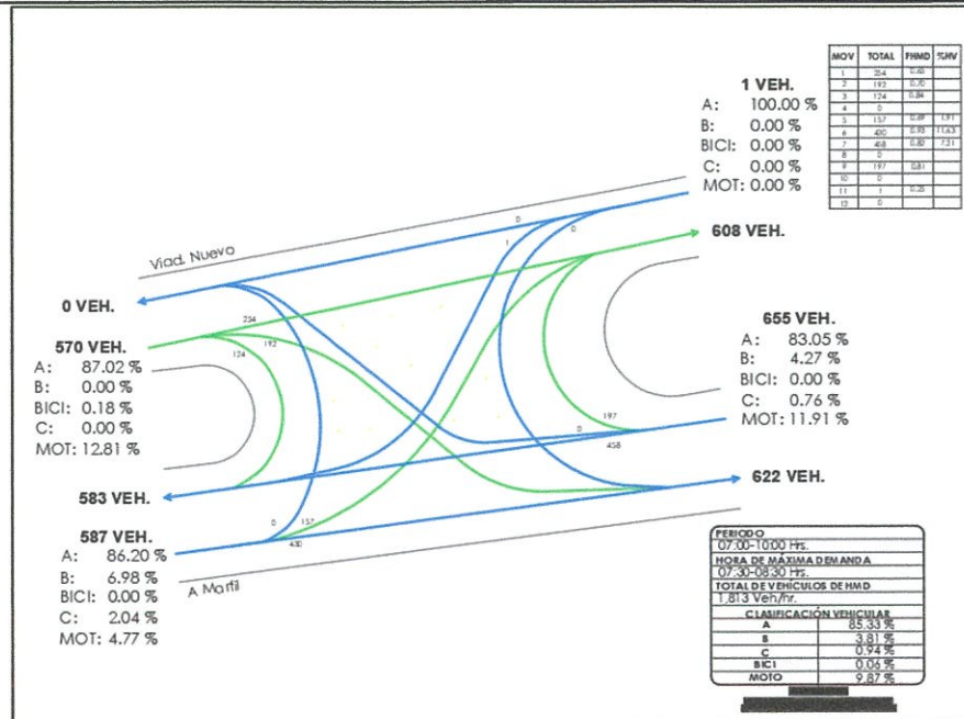
Ilustración 05 Volúmenes de tránsito vehicular y ciclista Carr. Marfil – Viaducto nuevo (turno mañana)
