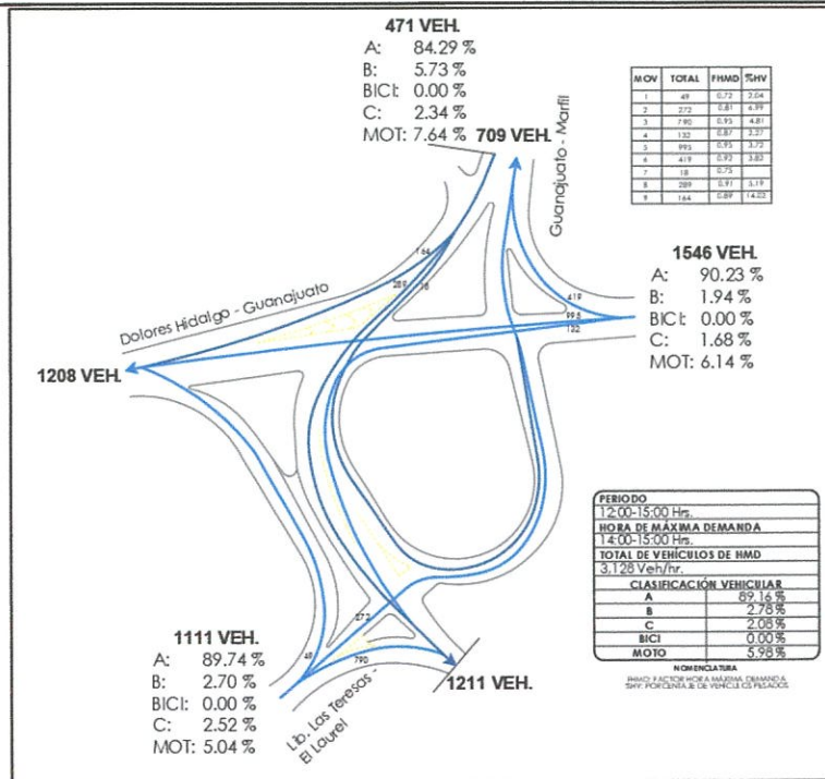
Ilustración 21 Volúmenes de tránsito vehicular y ciclista Glorieta Marfil – Carr. Guanajuato – Silao (turno medio día) Fuente: Elaboración propia
