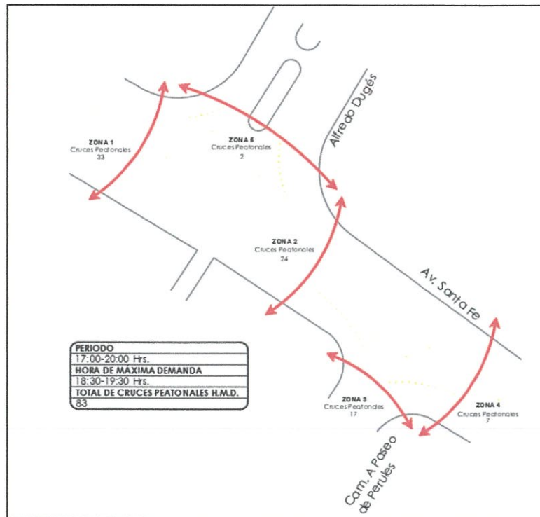
Ilustración 36 Volúmenes peatonales Avenida Santa Fe – calle Alfredo Dugés (turno tarde)
