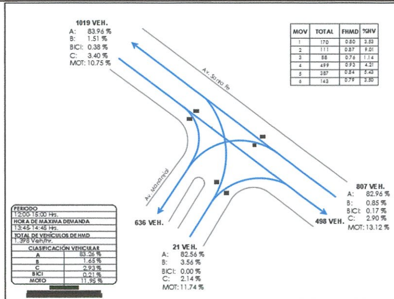
Ilustración 25 Volúmenes de tránsito vehicular y ciclista Carr. puentecillas - Manantial (turno medio día)
