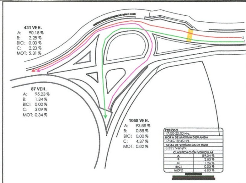
Ilustración 25 Volúmenes de tránsito vehicular y ciclista Carretera Guanajuato – Juventino Rosas (curvas peligrosas) (turno tarde)
