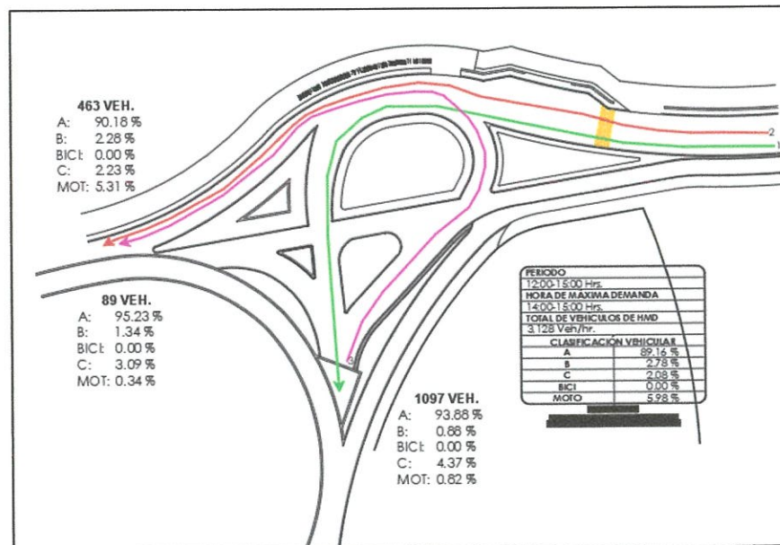
Ilustración 24 Volúmenes de tránsito vehicular y ciclista Carretera Guanajuato – Juventino Rosas (curvas peligrosas) (turno medio día) Fuente: Elaboración propia
