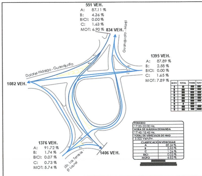
Ilustración 22 Volúmenes de tránsito vehicular y ciclista Glorieta Marfil – Carr. Guanajuato - Silao (turno tarde) Fuente: Elaboración propia
