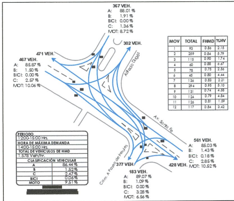
Ilustración 15 Volúmenes de tránsito vehicular y ciclista Av. Santa Fe – Calle Alfredo Dugés (turno medio día) Fuente: Elaboración propia
