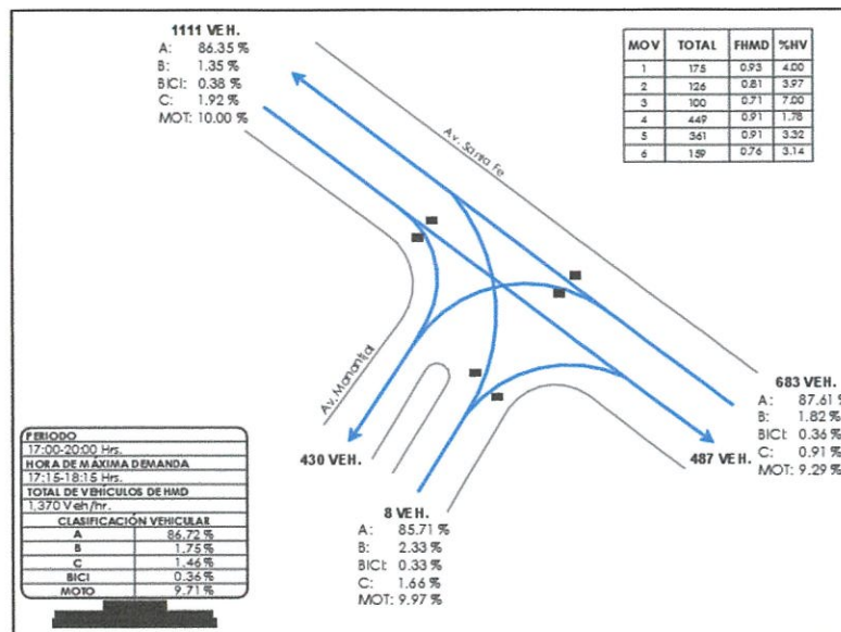
Ilustración 25 Volúmenes de tránsito vehicular y ciclista Carr. puentecillas - Manantial (turno tarde)
