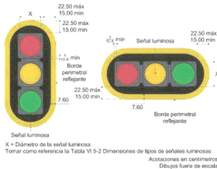
Figura VI.5-10 Semáforo general vertical y horizontal para vehículos
