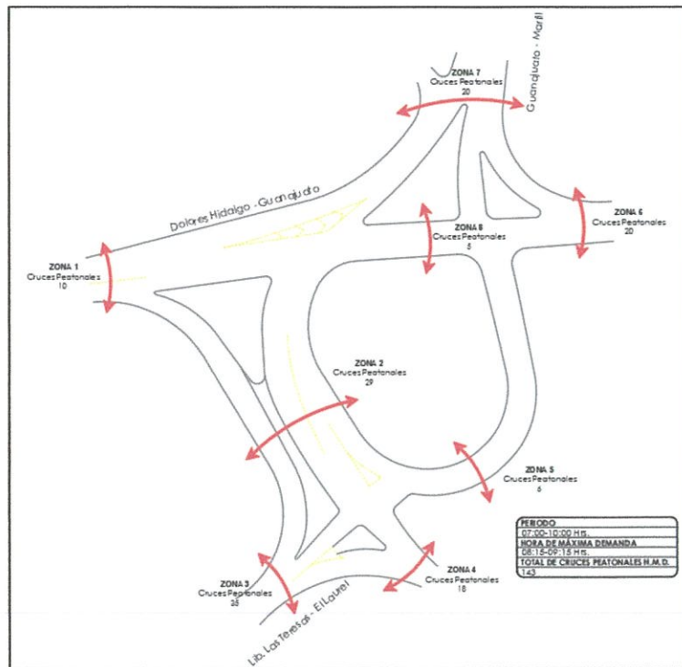
Ilustración 40 Volúmenes peatonales Glorieta Marfil – Carr. Guanajuato Silao (turno mañana)
