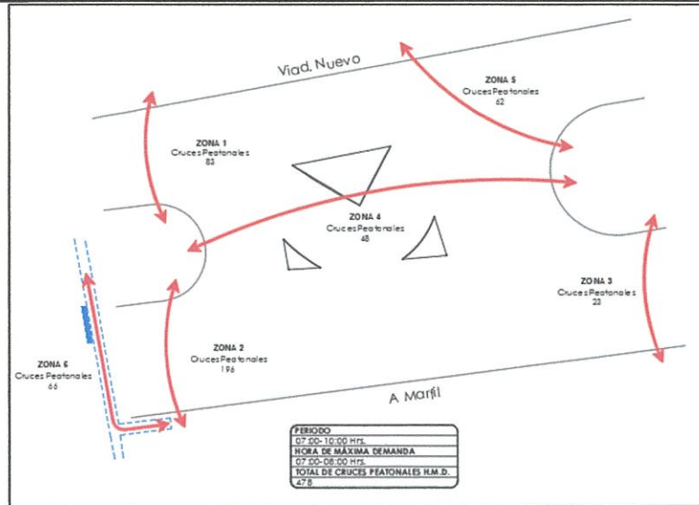
Ilustración 26 Volúmenes peatonales Carr. Marfil – Viaducto Nuevo (turno mañana)
