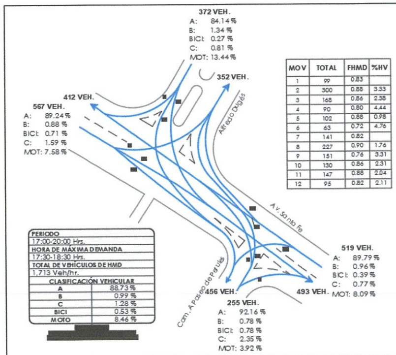
Ilustración 16 Volúmenes de tránsito vehicular y ciclista Av. Santa Fe – Alfredo Dugés (turno tarde) Fuente: Elaboración propia
