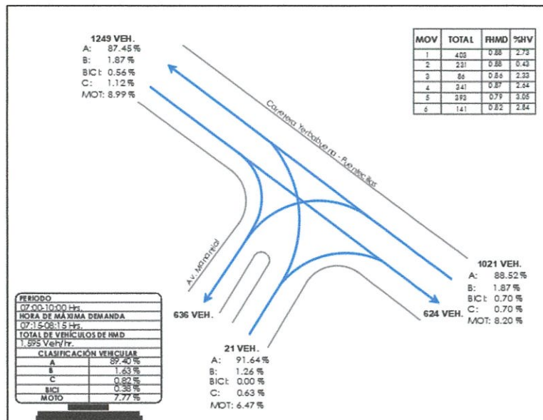
Ilustración 25 Volúmenes de tránsito vehicular y ciclista Carr. puentecillas - Manantial (turno mañana)
