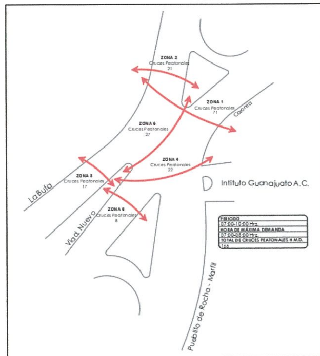
Ilustración 29 Volúmenes peatonales Carr. Marfil - Calle La Bufa (turno mañana) Fuente: Elaboración propia
