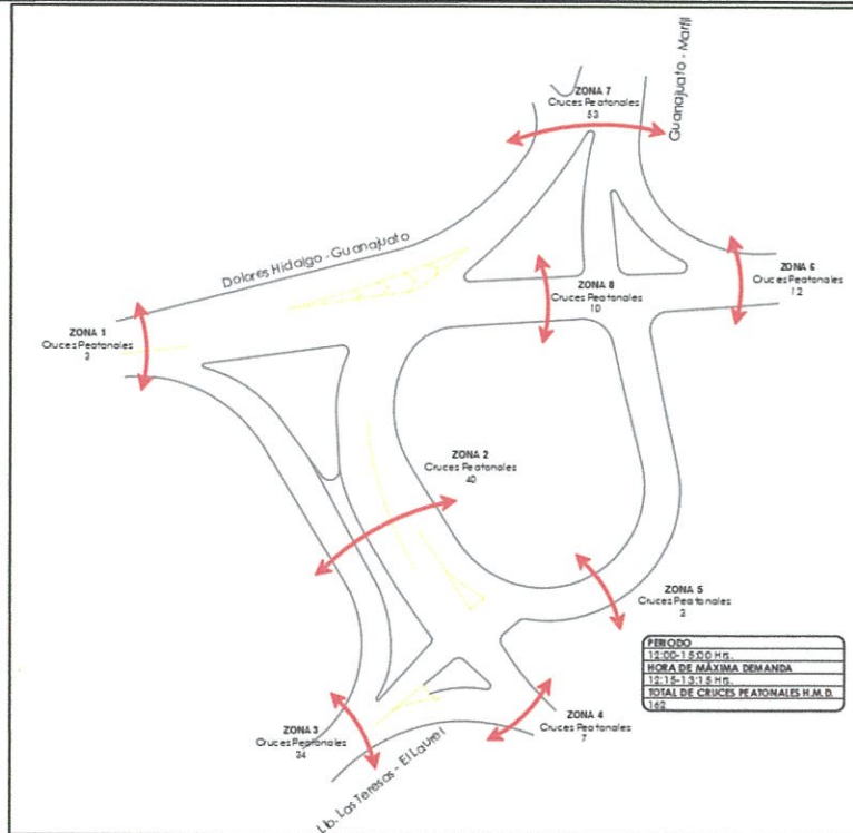
Ilustración 41 Volúmenes peatonales Glorieta Marfil – Carr. Guanajuato Silao (turno medio día)
