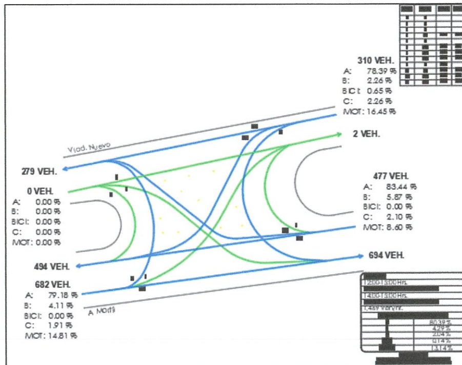
Ilustración 06 Volúmenes de tránsito vehicular y ciclista Carr. Marfil – Viaducto nuevo (turno medio día)
