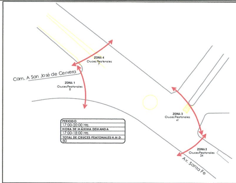
Ilustración 33 Volúmenes peatonales Avenida Santa Fe – Camino a Cervera (turno tarde)
