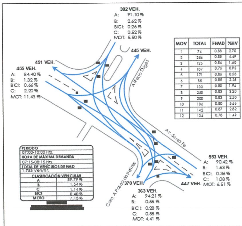
Ilustración 14 Volúmenes de tránsito vehicular y ciclista Av. Santa Fe – Calle Alfredo Dugés (turno mañana)
