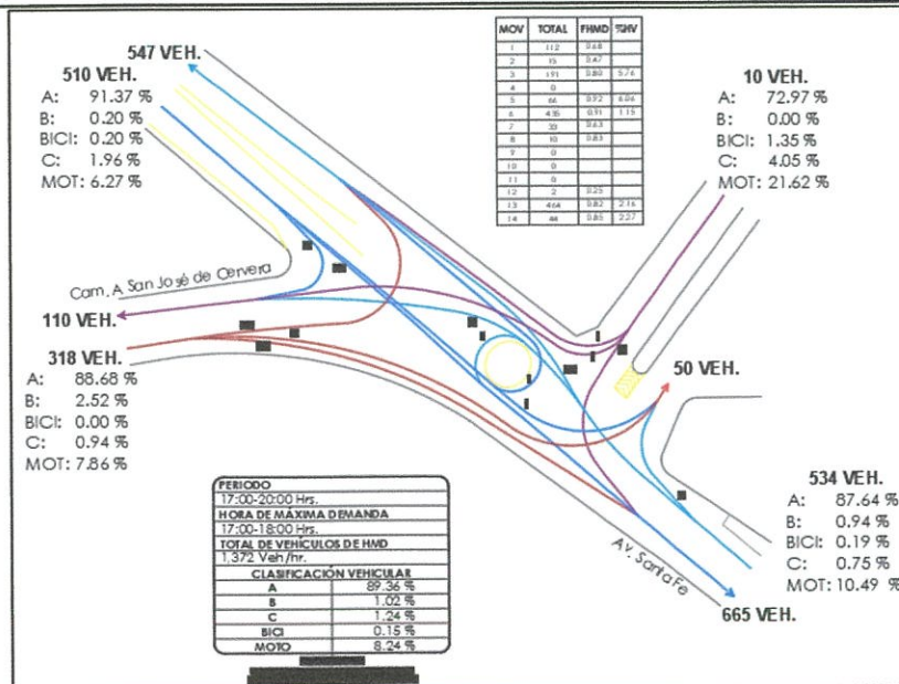
Ilustración 13 Volúmenes de tránsito vehicular y ciclista Av. Santa Fe – Camino a Cervera (turno tarde)
