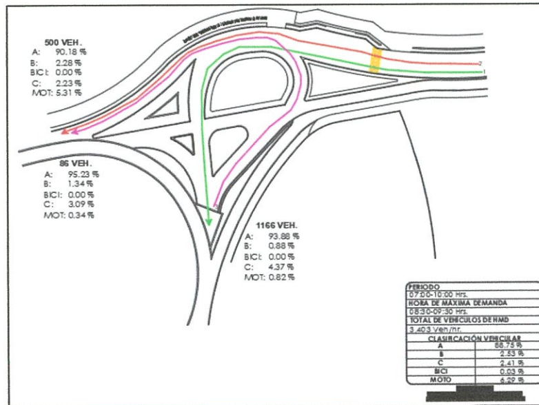
Ilustración 23 Volúmenes de tránsito vehicular y ciclista Carretera Guanajuato – Juventino Rosas (curvas peligrosas) (turno mañana) Fuente: Elaboración propia
