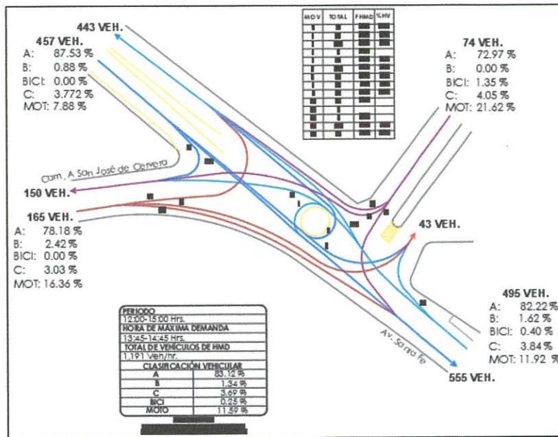
Ilustración 12 Volúmenes de tránsito vehicular y ciclista Av. Santa Fe – Camino a Cervera (turno medio día)
