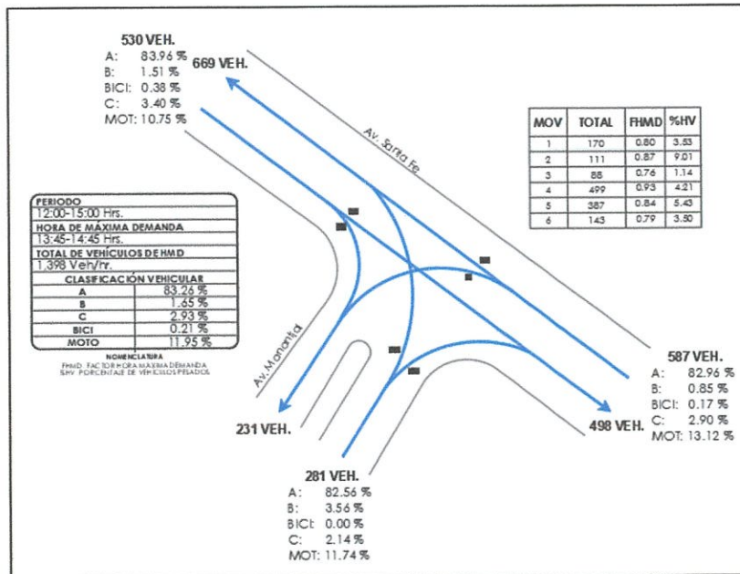
Ilustración 18 Volúmenes de tránsito vehicular y ciclista Av. Santa Fe – Manantial (turno medio día)
