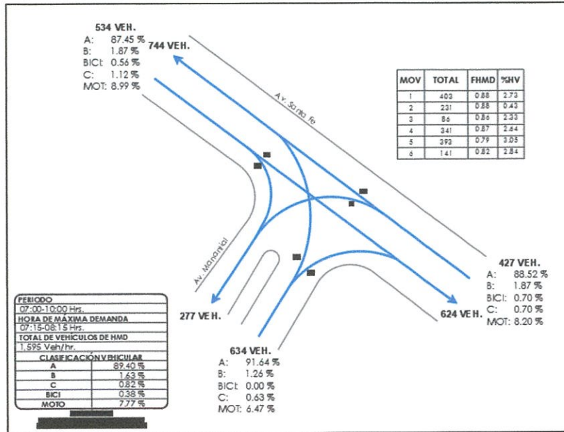
Ilustración 17 Volúmenes de tránsito vehicular y ciclista Av. Santa Fe – Manantial (turno mañana)
