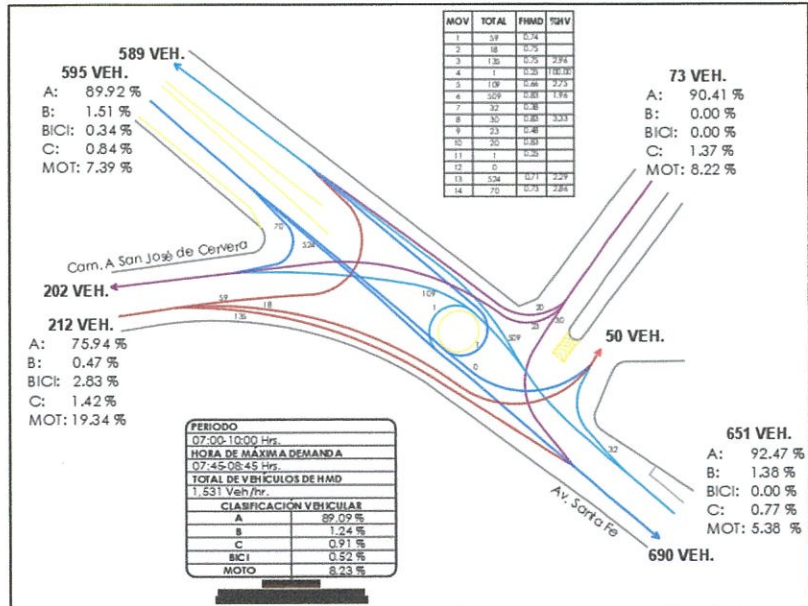
Ilustración 11 Volúmenes de tránsito vehicular y ciclista Av. Santa Fe – Camino a Cervera (turno mañana)
