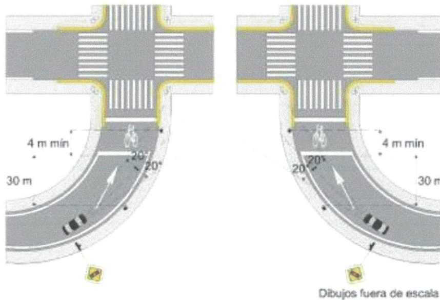
Figura VI.5-12 Ubicación de semáforo en curva horizontal
