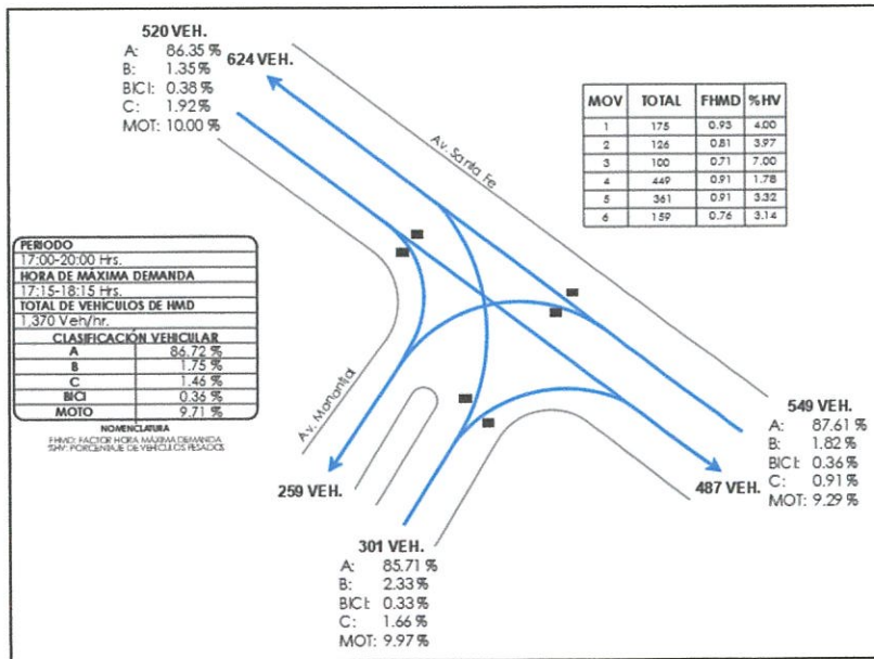
Ilustración 19 Volúmenes de tránsito vehicular y ciclista Av. Santa Fe – Manantial (turno tarde)
