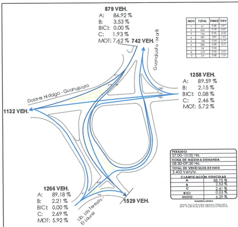
Ilustración 20 Volúmenes de tránsito vehicular y ciclista Glorieta Marfil – Carr. Guanajuato - Silao (turno mañana)
