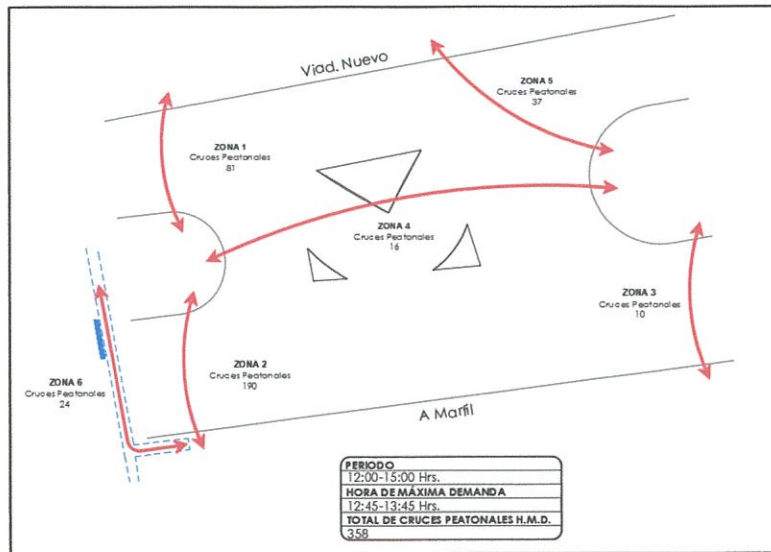
Ilustración 27 Volúmenes peatonales Carr. Marfil – Viaducto Nuevo (turno medio día)
