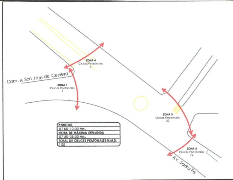
Ilustración 31 Volúmenes peatonales Avenida Santa Fe – Camino a Cervera (turno mañana) Fuente: Elaboración propia
